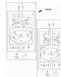
C.1, ETV-013068, диск для разбрасывания удобрения по краю поля TS 5-9 , 1
