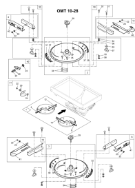
B.5, ETV-013065, распределяющий диск OMT 10-28 , 1
