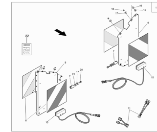
N.4, ETV-013104, габаритное освещение передн. для насадки L1000 , 1
