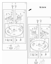
C.2, ETV-013069, диск для разбрасывания удобрения по краю поля TS 10-14 , 1
