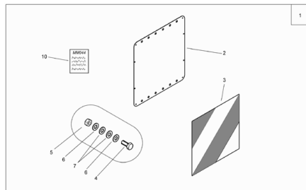
N.5, ETV-013105, Warntafeln für Frankreich ab Bj.2009 !, 1
