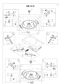
B.2, ETB-013062, распределяющий диск OM 10-16 , 1
