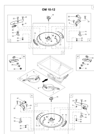
B.1, ETB-013061, распределяющий диск OM 10-12 , 1
