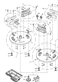
C.4, ETV-013071, диск для разбрасывания удобрения по краю поля TS 4 , 1
