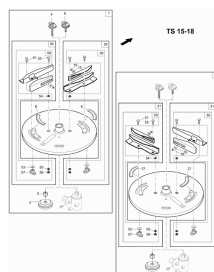
C.3, ETV-013070, диск для разбрасывания удобрения по краю поля TS 15-18 , 1
