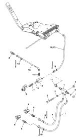
J.2, ETV-013090, гидравл.управление одинарных заслонок со стопорным устройством , 1
