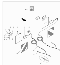
N.6, ETV-013106, освещение передн. для насадки L800 от года выпуска 2009 !, 1
