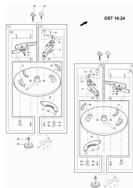
B.6, ETV-013066, Streuscheibe OST 10-24, 1
