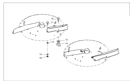
B10, ETV-013067, Базовые разбрасывающие лопатки, 1
