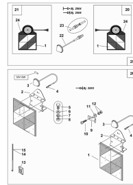
N.2, ETV-013102, габаритные фонари , 1
